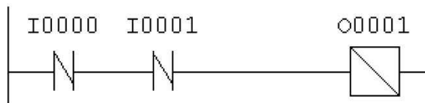
NOR ( NÃO OU )
