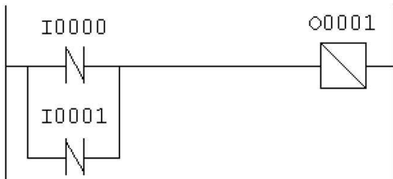
NAND ( NÃO E )
